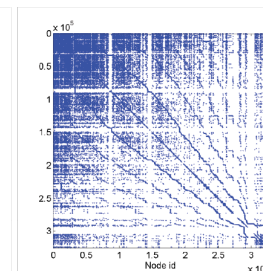
(l) www
