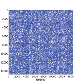
(g) IMDB
