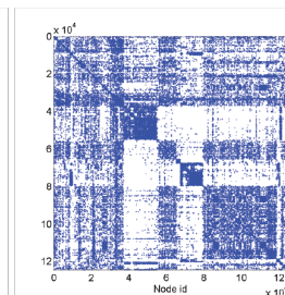
(k) internet
