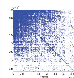
(j) enron
