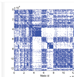
(k) internet
