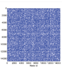
(g) IMDB
