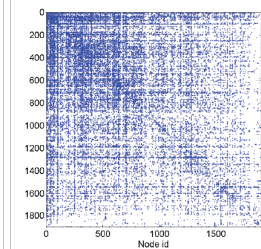
(d) UCirvine
