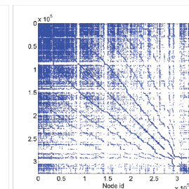
(l) www
