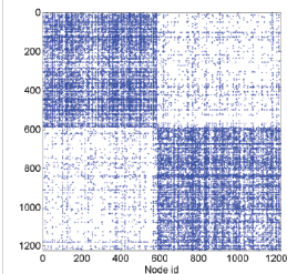
(b) polblogs
