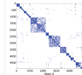
(f) USpower
