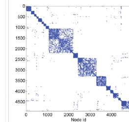
(f) USpower
